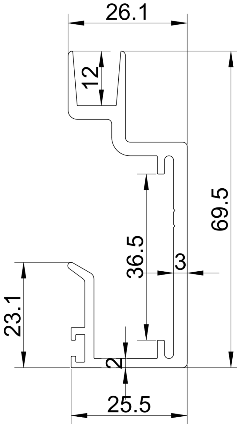
Rysunek profilu aluminiowego
